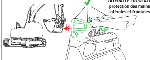
SPECIALE MANIGLIA DI GUIDA CON PROTEZIONI poignée spéciale
